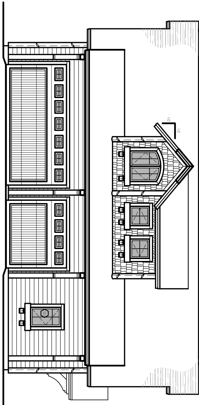
FRONT ELEVATION SCALE: 1/8" = 1'-0"
